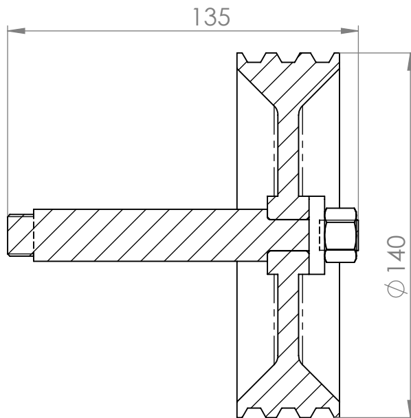
PRZEKRÓJ A-A
